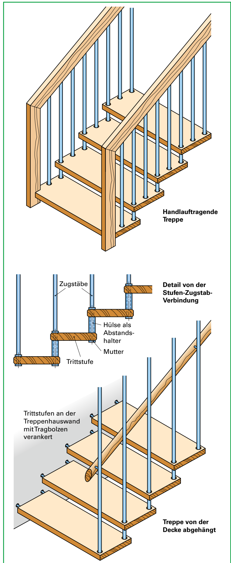
Bild 26/1: Abgehängte Treppen
