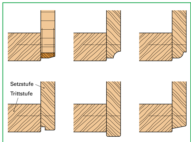
Bild 21/2: Anschluss der Setzstufe an die Trittstufe
