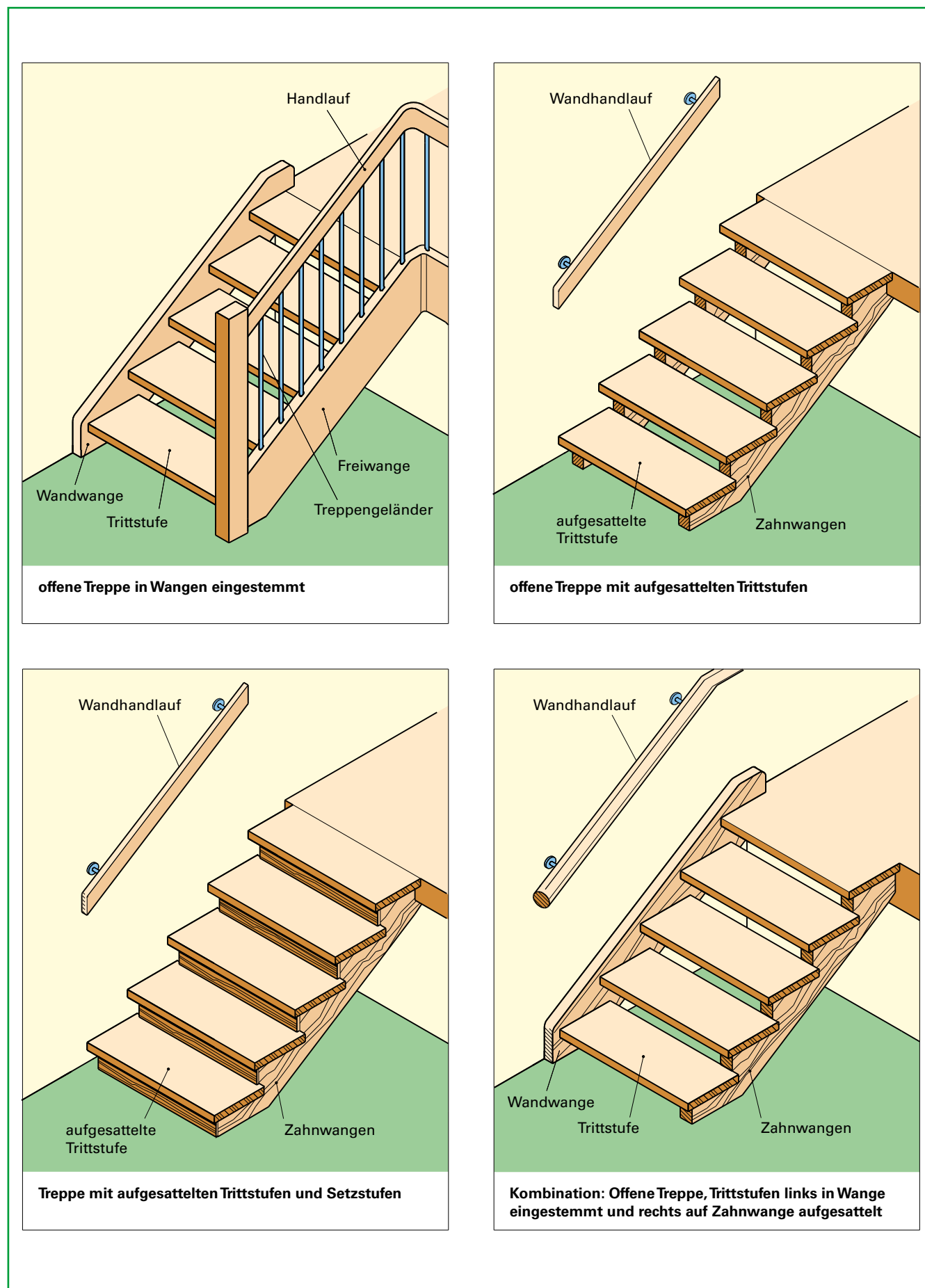
Bild 23/1: Weitere traditionell konstruierte Holztreppen
